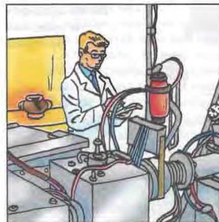
Радиоуглеродный метод датировки источников
